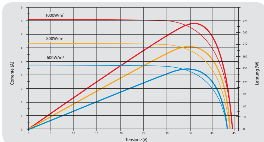
Curva corrente/tensione e potenza/tensione (260W)
