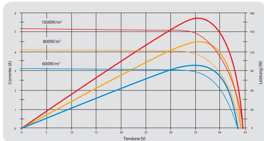
Curva corrente/tensione e potenza/tensione (175W)
